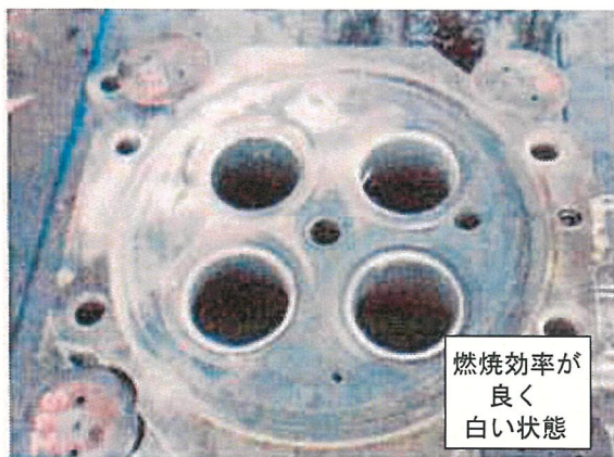
換気口のカーボン も簡単に剥がれ 落ちる状態
