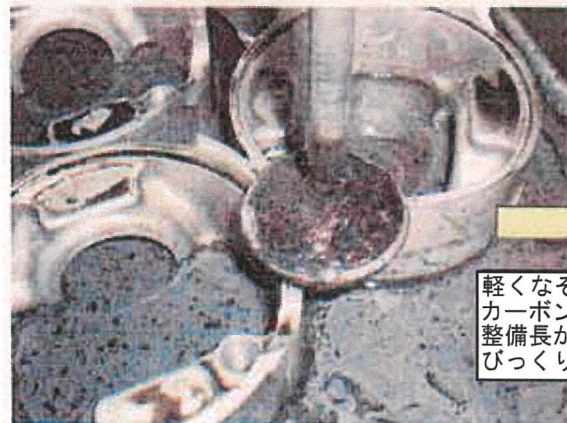
簡単にカーボンが 剥がれ落ちる状態
